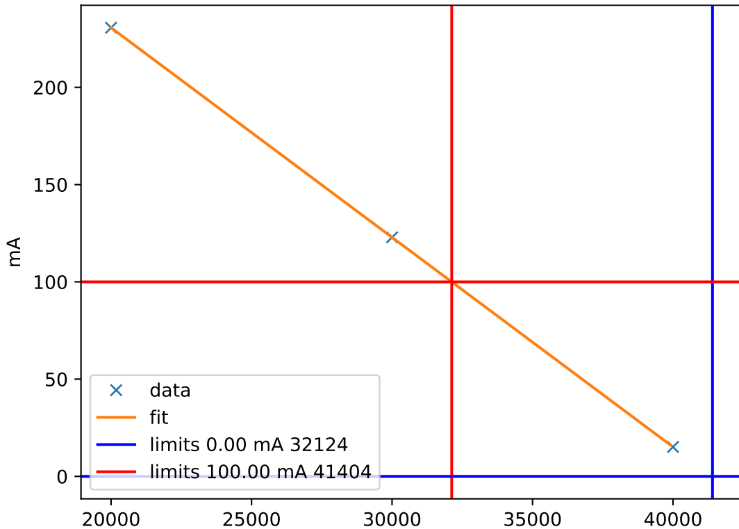
csense_15v
