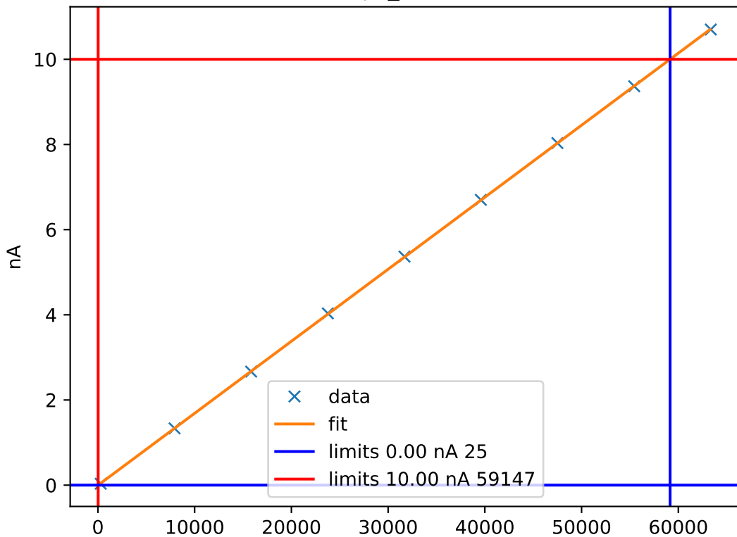
hvps_csense
